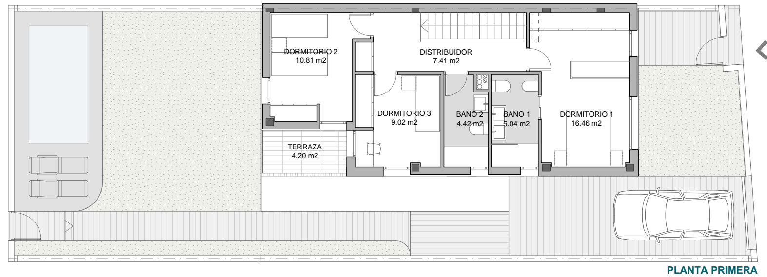
PLANTA PRIMERA
